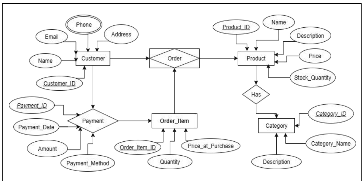
Fig: ER Diagram of Online Store
